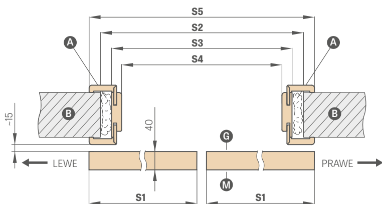
SP2N (Vorderseite)
