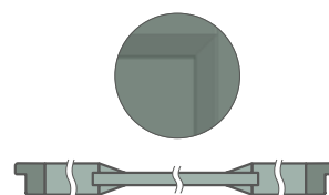
WERBENA 1, 2, 3 flache Schrägleiste an der 16 mm Platte
