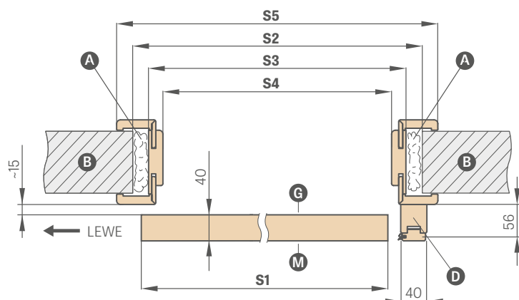
SP1Nz oder SP1Nb (links Vorderseite)
